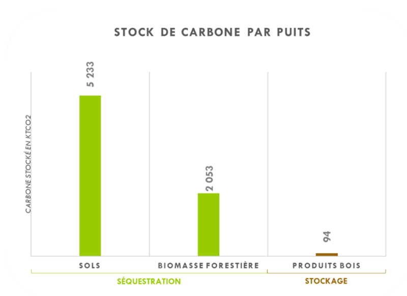
Graphique 25 : Stock de carbone par puits – CC Gartempe – Saint-Pardoux
