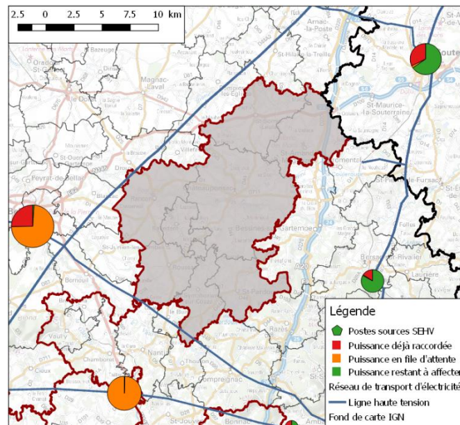
Figure 5 : Disponibilité affichée dans le S3RENR
